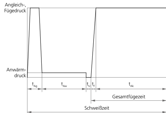
Abbildung C.2: Prozessschritte des beheizten Werkzeugstumpfschweißens gemäß DVS 2207-1.
